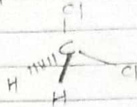
Dichloromethane ( \text{CH}_2\text{Cl}_2 )
